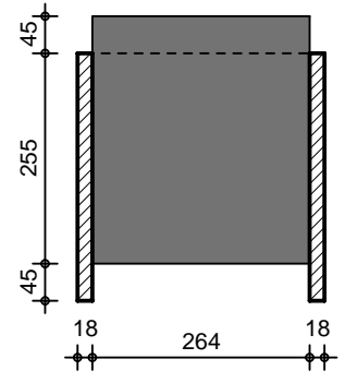
VUE EN COUPE AA
