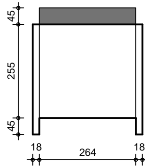
VUE LATERALE
