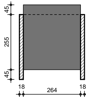
VUE EN COUPE AA
