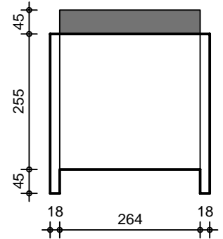
VUE LATÉRALE
