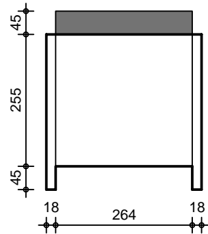
VUE LATÉRALE
